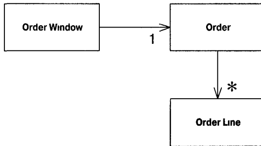
Рис. 12.9. Классы окна заказа и заказа
