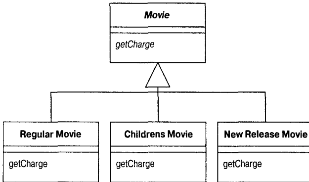
Рис. 1.14. Применение наследования для Movie
