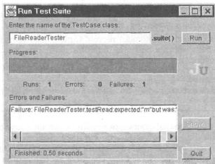
Рис. 4.2. Графический интерфейс пользователя в JUnit
